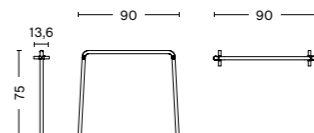
PALISSADE MIDDLE LEG Width 90 cm Depth 13,6 cm Heigth 75 cm
